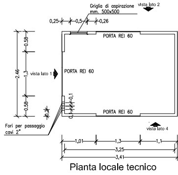
Pianta locale tecnico
