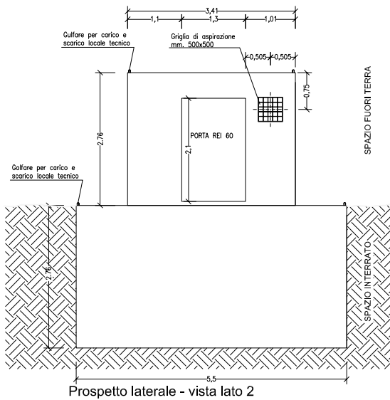
Prospetto laterale - vista lato 2
