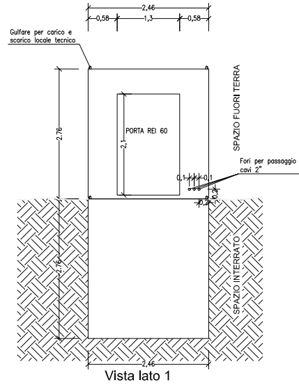
Vista lato 1
