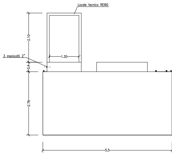
Prospetto laterale - vista lato 1
