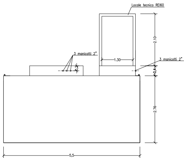
Prospetto laterale - vista lato 3
